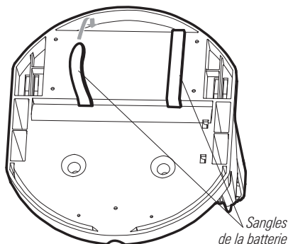
Fixation des sangles de la batterie
