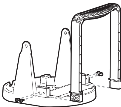
Installation de la poignée sur le socle
